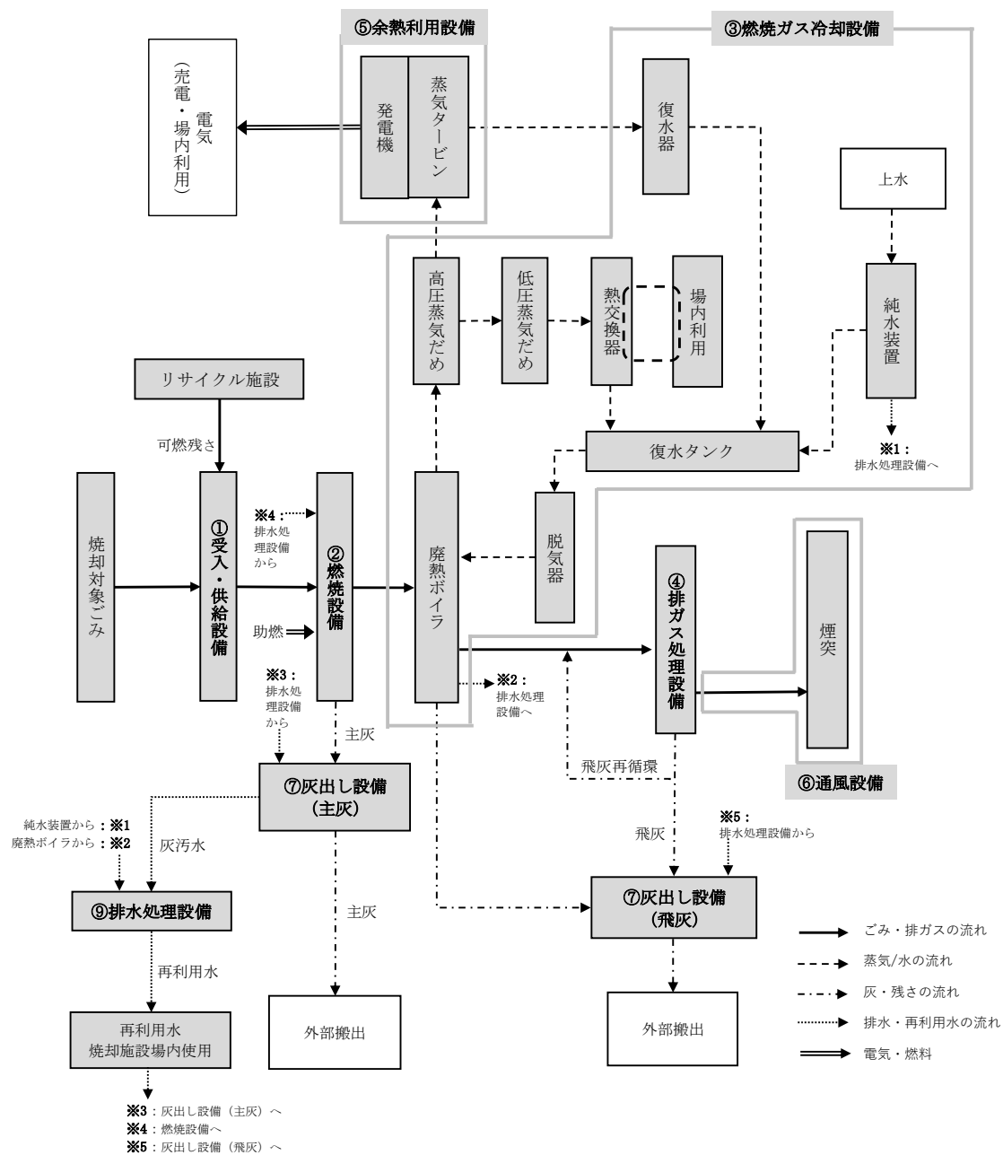
図1 エネルギー回収推進施設 全体処理フロー（案）（参考）
