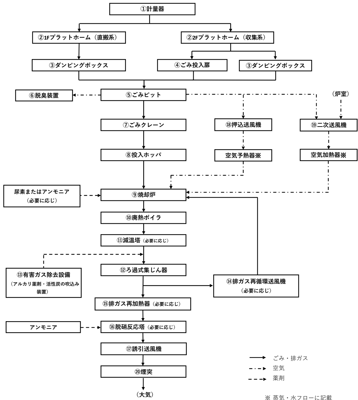
図2 ごみ・排ガスフロー（参考）
