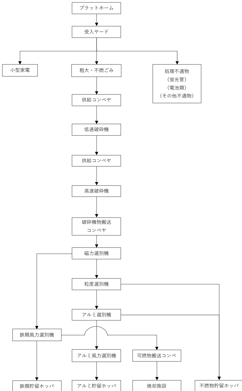
図1 粗大・不燃ごみ処理フロー (低速破砕機+高速破砕機の1系列の場合)
