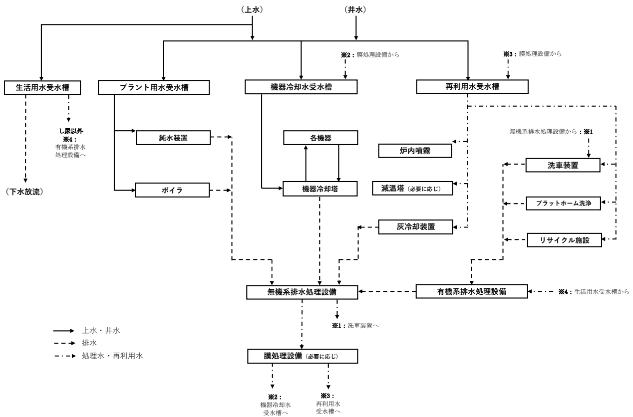
図4 給水・排水フロー (参考)
