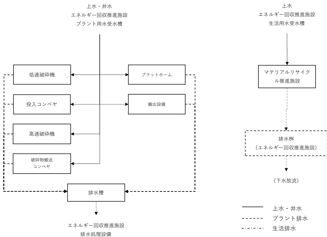
図4 給排水フロー
