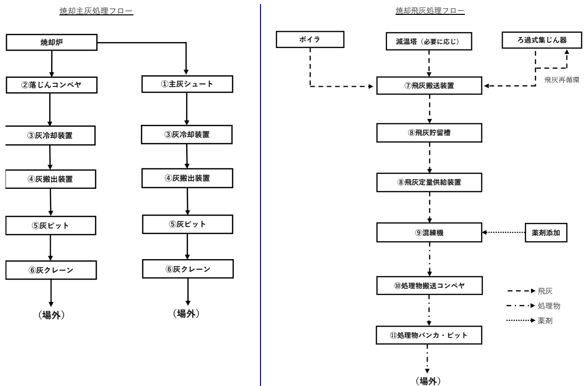
図5 主灰・飛灰処理フロー (参考)
