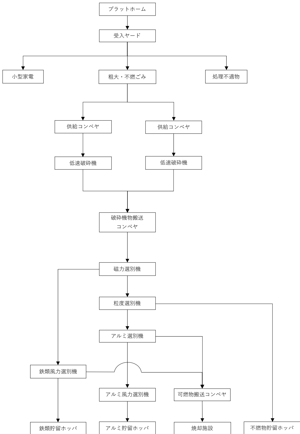
図2 粗大・不燃ごみ処理フロー（低速破碎機のための2系列の場合）
