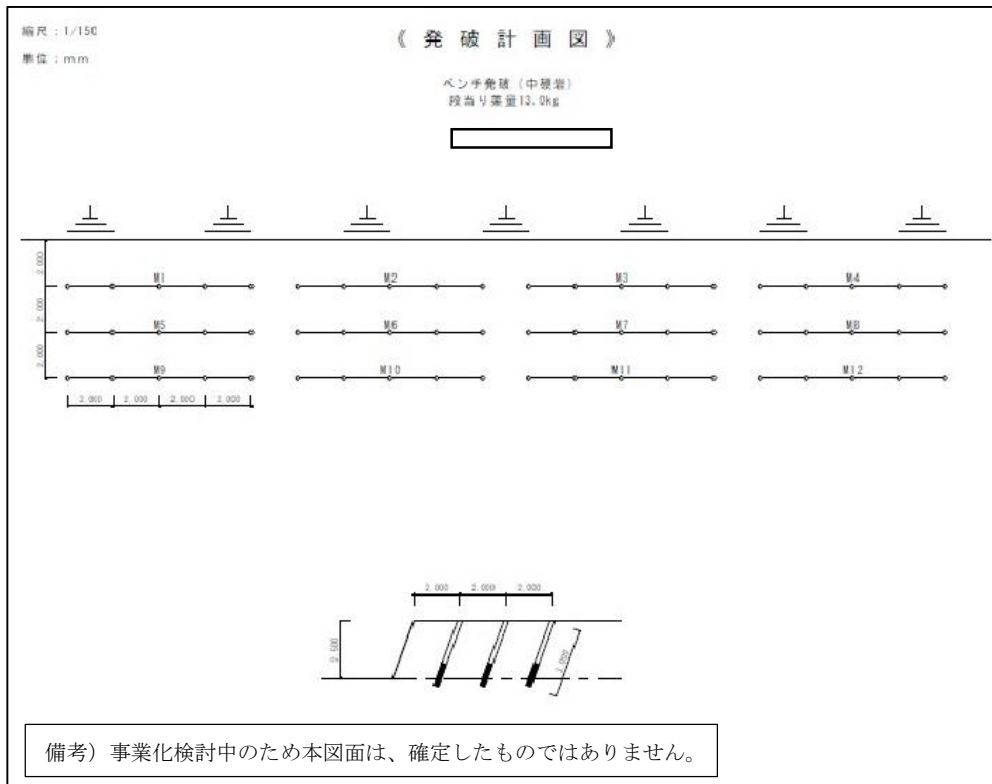
図 7. 5 - 8 発破計画図
