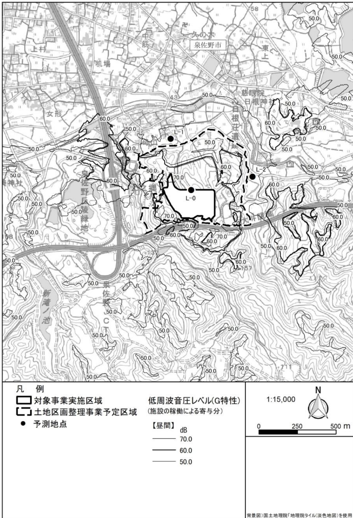
図 7. 5-5 (1) エネルギー回収推進施設等の稼働による低周波音の予測結果 (昼間)
