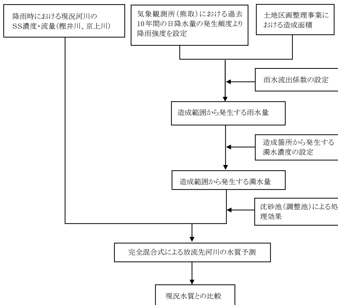
図 7. 2-12 予測フロー
