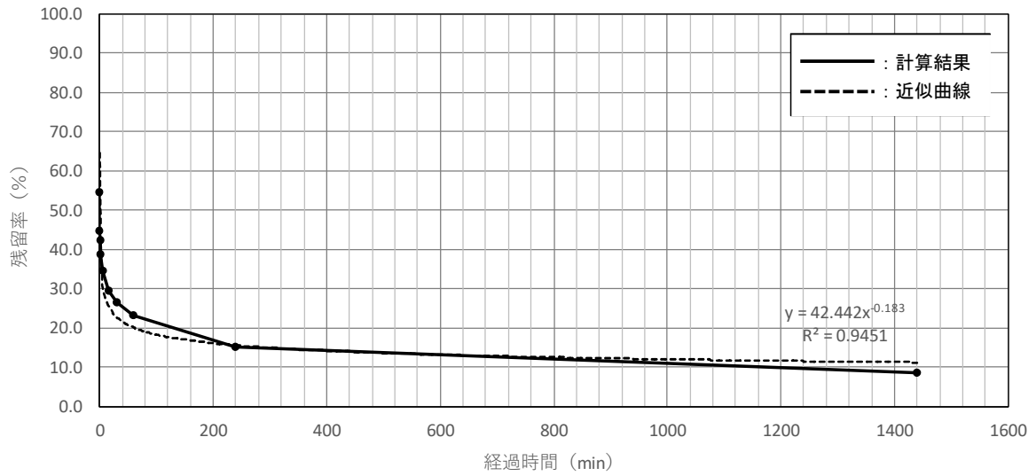
図 7. 2-8 経過時間と残留率の関係 (NO. 5・P-1)
